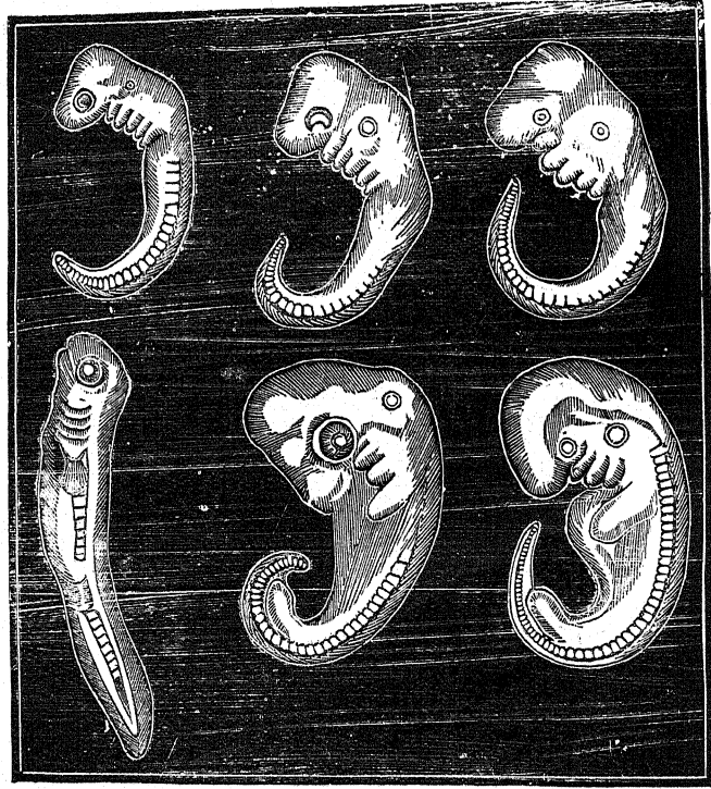
चित्र ६३—अणू का विकास
